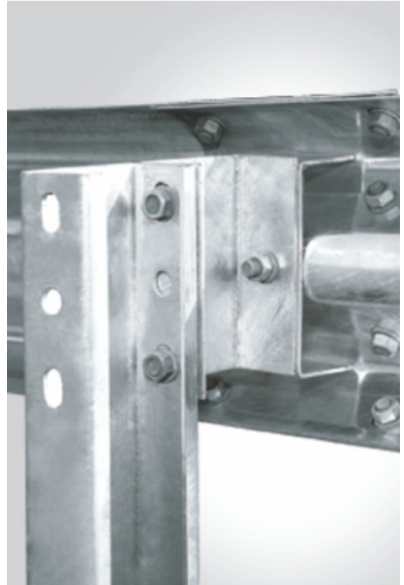
Sistema de acoplamento das peças por parafusos. Facilita a manutenção e desvios de emergência.
